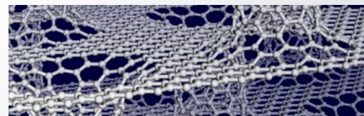
Графен
