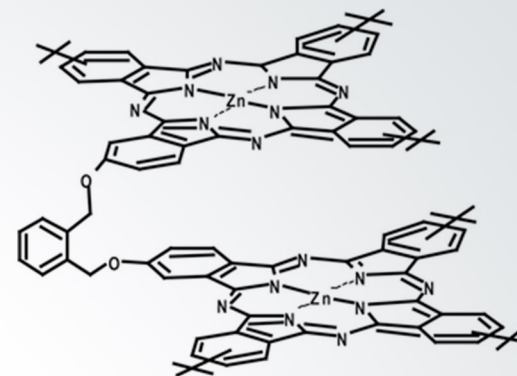
Фталоцианин
