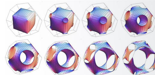
Поверхность Ферми
