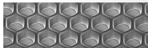
Сапфир
